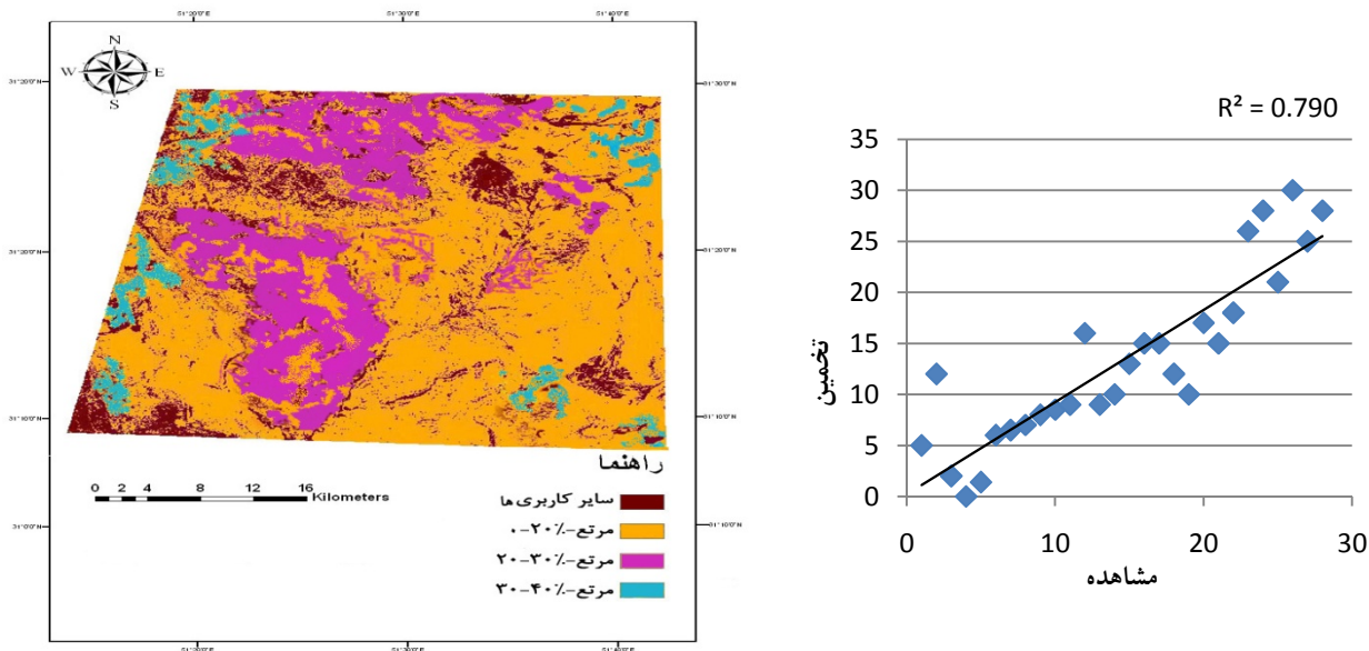
شکل ۳. نقشه درصد پوشش گیاهی مراتع سال ۱۳۸۳ و نمودار تعیین دقت نقشه به روش Cross Validation
