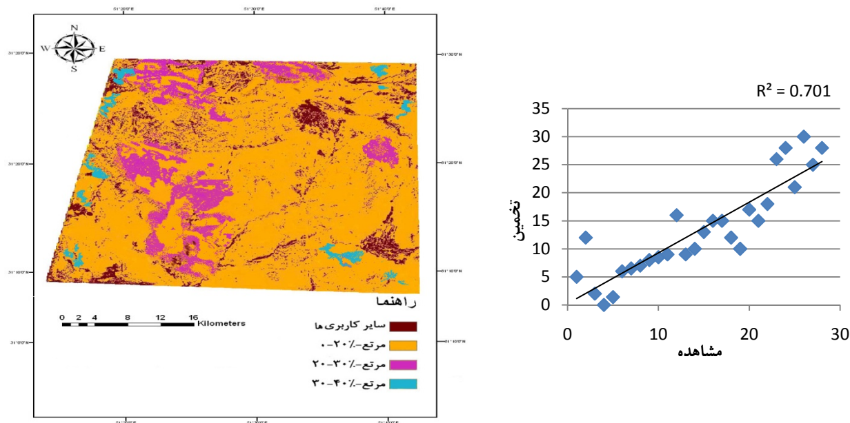
شکل ۴. نقشه درصد پوشش گیاهی مراتع سال ۱۳۸۸ و نمودار تعیین دقت نقشه به روش Cross Validation
