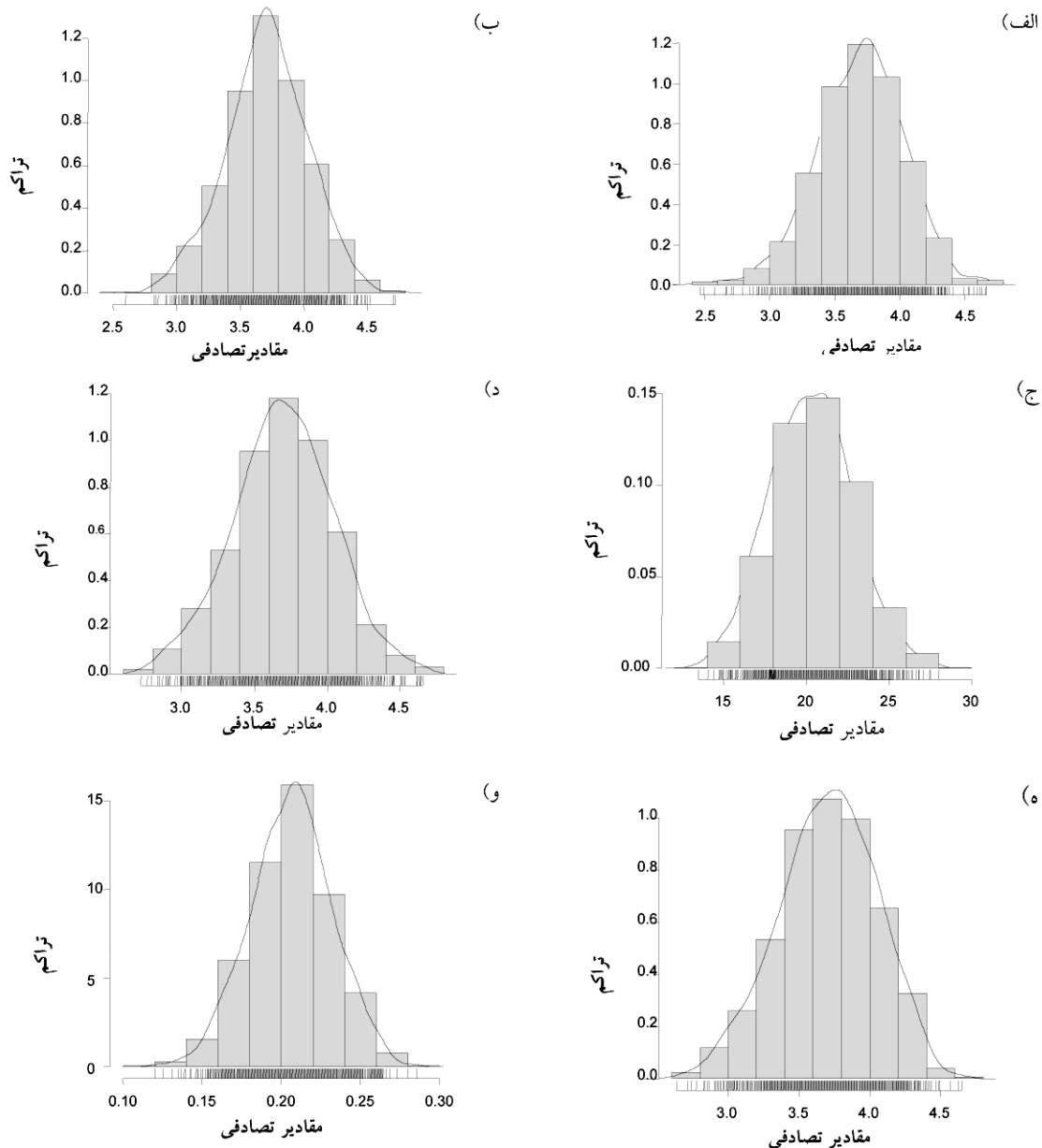
شکل ۴. توزیع ضریب تغییرات عدم قطعیت به روش بوت‌استرپ برای شاخص‌های اکولوژیک آبخیز چهل‌چای
