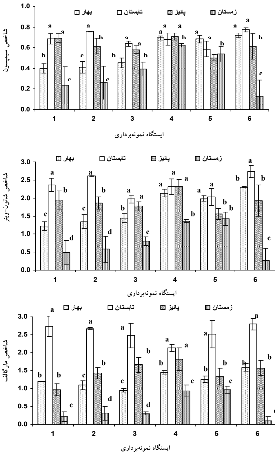
شکل ۲. شاخص‌های تنوع سیمپسون، شانون-وینر، و مارگالف فیتوپلانکتون‌های دریاچه سد حنا در ایستگاه‌های نمونه‌برداری و فصول مختلف. میانگین‌های دارای حداقل یک حرف مشابه در هر ایستگاه از نظر آماری با آزمون دانکن باهم اختلاف معنی‌داری ندارند ( P > 0.05 ).
