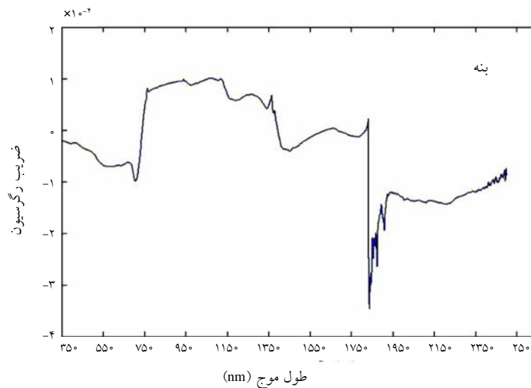
شکل ۲. نمودار ضرایب رگرسیون حاصل از مدل PLS در طول موج‌های مختلف برای LAI3D
