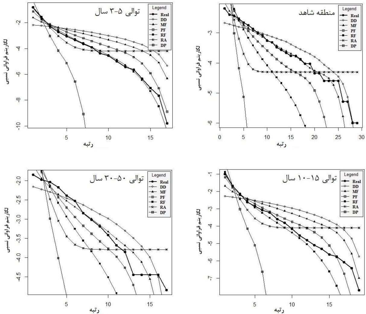
شکل ۴. منحنی توزیع فراوانی مدل‌های آشبان اکولوژیک در هر یک از مناطق مورد مطالعه؛ Real: منحنی داده‌های واقعی، DP: چیرگی پیش‌دست، RA: جورسازی تصادفی، RF: شکست تصادفی، PF: شکست توانی، MF: شکست مک‌آرتور و DD: زوال چیرگی
