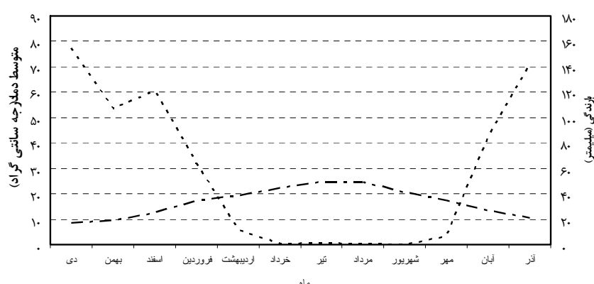
نمودار ۱. آبروترمیک شهرستان ایذه
