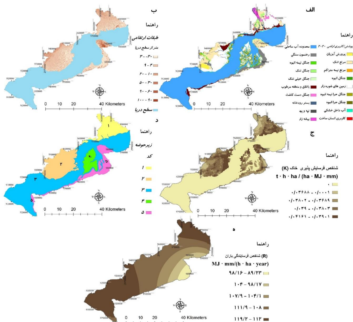
شکل ۲. داده های نقشه ای ورودی مدل InVEST SDR در محدوده مورد مطالعه: (الف) نقشه پوشش / کاربری زمین، (ب) مدل رقومی ارتفاع، (ج) شاخص فرسایش پذیری خاک (K)، (د) زیرحوضه های آبخیز، (ه) شاخص فرسایش پاران (R)
