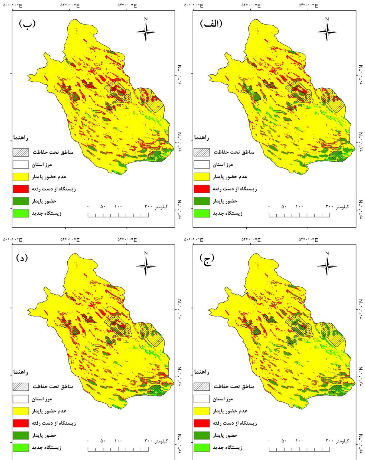
شکل ۳. نقشه‌های پیش‌بینی زیستگاه کل‌وز تحت سناریوهای اقلیمی و دو مدل گردش عمومی
