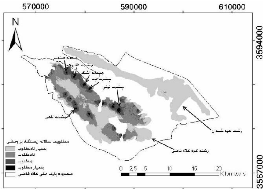
شکل ۲. نقشه مطلوبیت سالانه زیستگاه بز وحشی در چهار طبقه مطلوبیت در محدوده زیستگاه آن در پارک ملی کلاه‌قازی
