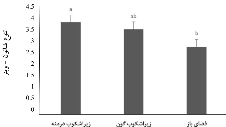
شکل ۷. مقایسه شاخص تنوع شانون-وینر در زیراشکوب درمنه، زیراشکوب گون و فضای باز
