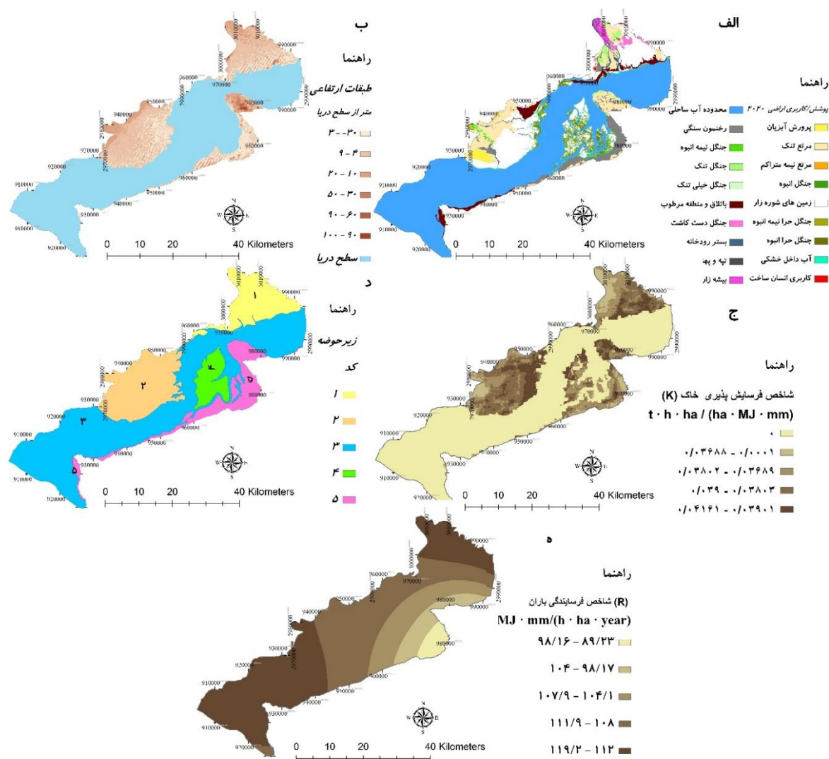
شکل ۲. داده های نقشه ای ورودی مدل InVEST SDR در محدوده مورد مطالعه: (الف) نقشه پوشش / کاربری زمین، (ب) مدل رقومی ارتفاع، (ج) شاخص فرسایش پذیری خاک (K)، (د) زیرحوضه های آبخیز، (ه) شاخص فرسایش پذیری باران (R)
